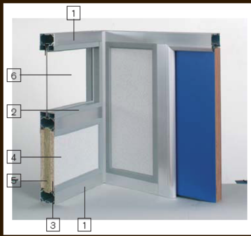
Сборка посредством скоб и эксцентриков
